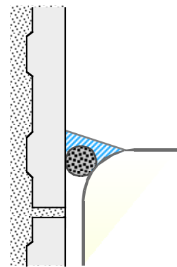
Figur 1 Fog mellan inbyggt badkar och vägg. Fogen utförs lutande för att underlätta avrinning och rengöring
